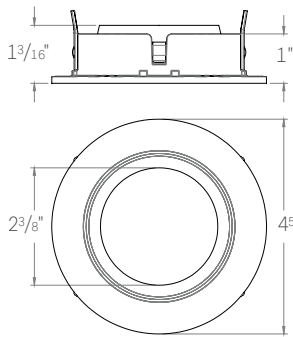
ED3-RFST ROUND STANDARD TRIM
