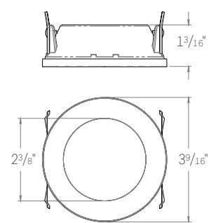
ED3-RFTL ROUND TRIMLESS
