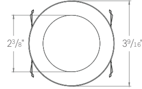
ED3-RFTL ROUND TRIMLESS
